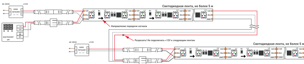
Рис. 1. Схема подключения ленты SPI-PFS-B60 с использованием SPI-контроллера с одним выходным портом и с использованием отдельных блоков питания
